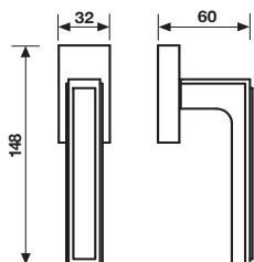
H 1056 F RS-41 Maniglia per finestra Window handle
