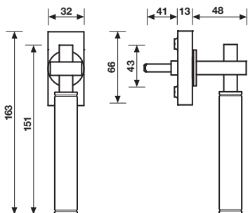
H 377 F RS-41 Movimento 4 scatti Movement 4 click positions
